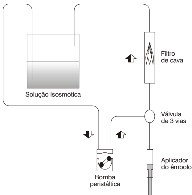
Figura 3 - Esquema mostrando o circuito utilizado para avaliação da eficácia in vitro dos filtros de veia cava Greenfield e Braile
